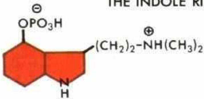
Psilocybin
