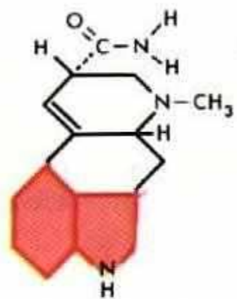
Isoergine
