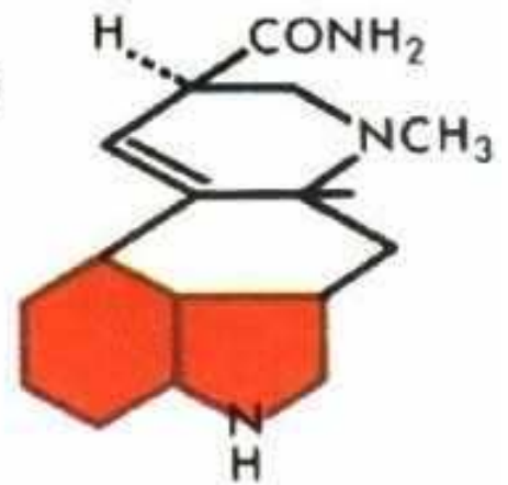
Ergine
