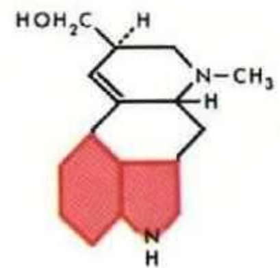
Lysergol
