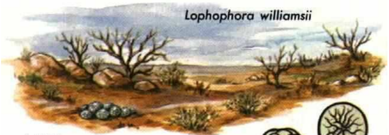
habitat
