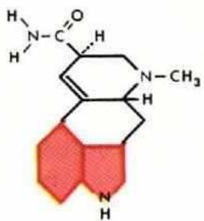
Ergine
