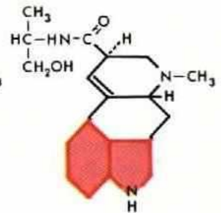
Ergometrine (Ergonovine)
