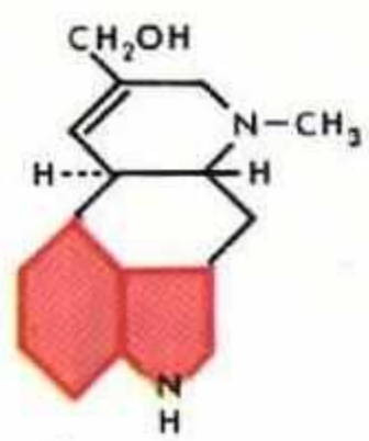
Elymoclavine
